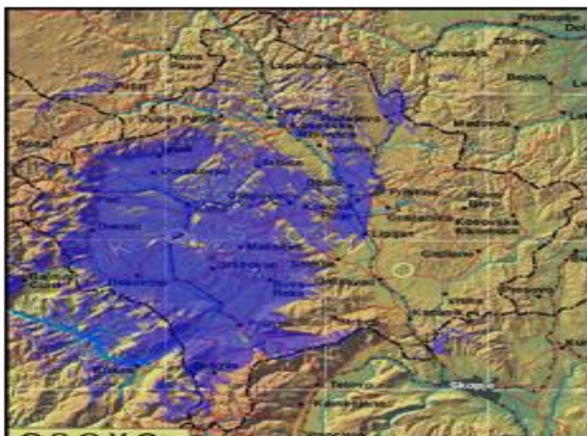
Korniza teknike / Figura 4 - Llogaritja e mbulimit të modifikuar (Cvilen -majtas, Zatriq-të djathtas). Cvilen : 49,7 dB \mu V (56 dB \mu V / m për pritjen fikse), Zatriq: 40 dB \mu V (56 dB \mu V / m për pranim fikse, 78 dB \mu V / m për pranim portativ, pranim mobil)
