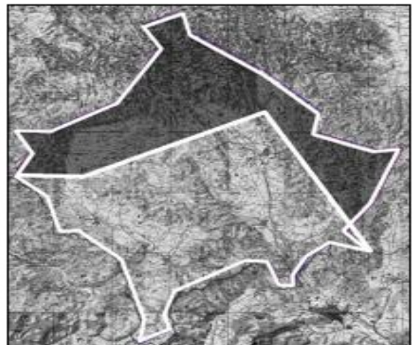
Korniza teknike/ Figura 6 dhe 7 - Forma e zonave të reja për transmetim dhe zonave të reja dhe të vjetra për transmetim – krahasimi (kufijtë e vendit me të zeza, kufijtë e zonës për transmetim me të bardha)
